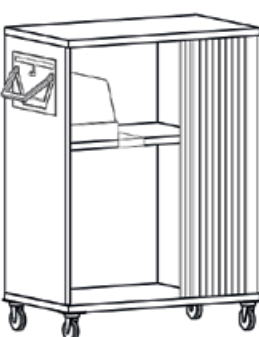
Mobilcontainer mit Posteinwurf und Postfach 743 x 463 x 1038
