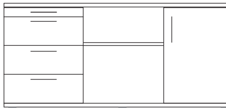
Schubladenelement Teilung 1/3/3/3 links CPU-Fach rechts 1200 x 600 x 570
