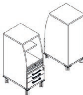
Personalcontainer 3 ohne ausklappbarem Oberboden und ohne Lenkgriffen 431 x 600 x 1038
