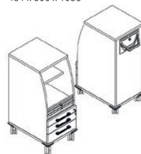
Personalcontainer 4 mit Briefeinwurf ohne ausklappbarem Oberboden und ohne Lenkgriffen 431 x 600 x 1038
