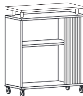
Mobilcontainer mit Abdeckplatte Distanzstücke 70mm ohne Überstand
